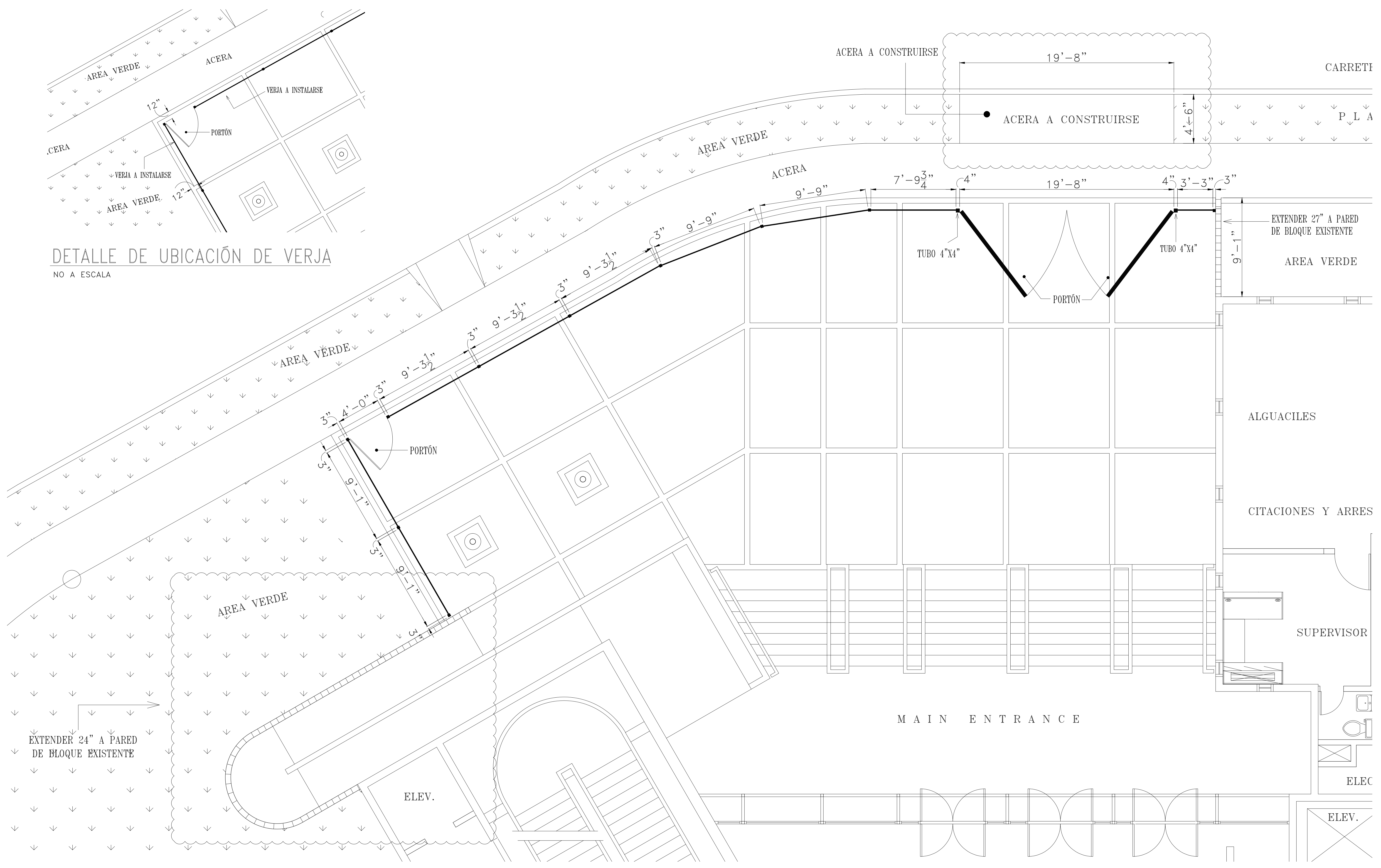
PLANTA DE PISO (VERJA FRONTAL) ESCALA: 1/4"=1'-0"
